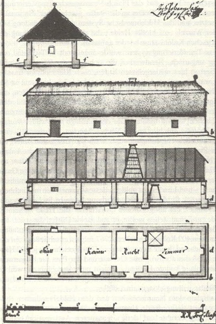
12. Plan eines Kolonistenhauses aus dem Jahre 1769
